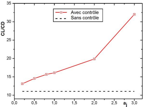
Fig. 5: Effet de l'amplitude de jet synthétique
