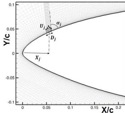
Fig.1: Représentation du jet synthétique
