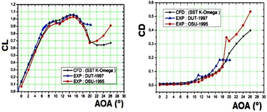
Fig. 3: Variation des coefficients de portance et de trainée en fonction de l'angle d'attaque
