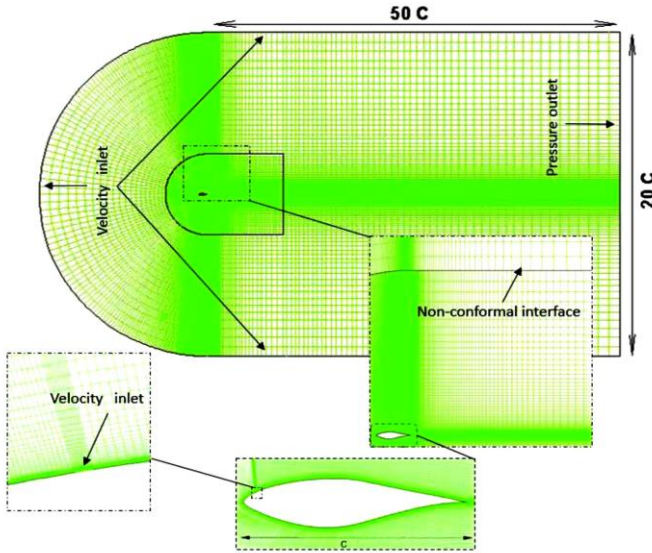
Fig. 2: Maillage et conditions aux limites
