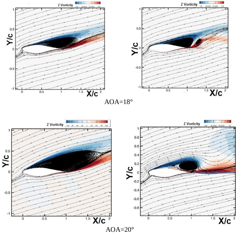
Fig. 8: Champs de vorticit  pour diff rents angles d'attaque.   gauche sans contr le et   droite avec contr le
