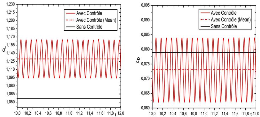
Fig. 6: Variation des coefficients C_L et C_D en fonction du temps
