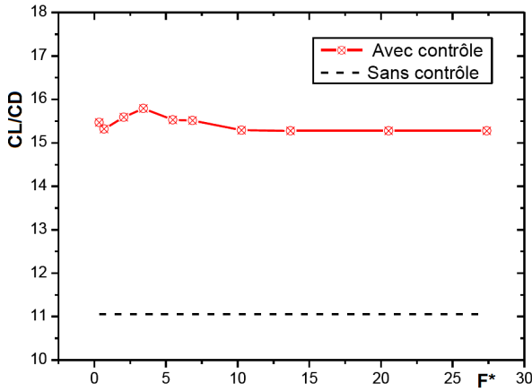
Fig. 7: Effet de la fréquence du jet
