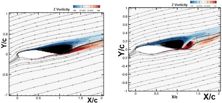
AOA= 15.1^\circ
