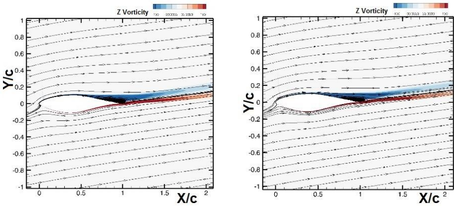
AOA= 10.1^\circ
