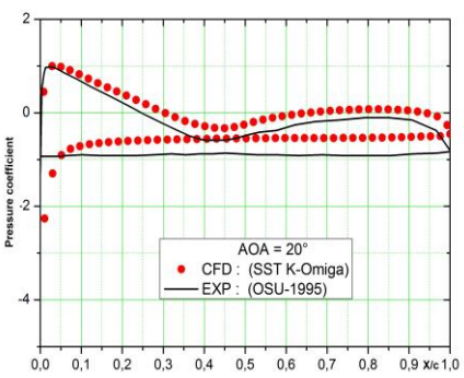
Fig. 4: Comparaison de la distribution de pression avec l'expérimental
